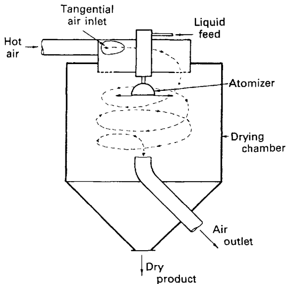
Fig. 26.11 Spray drier.
