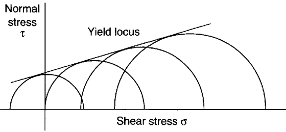
Fig. 14.3 Mohr diagram
